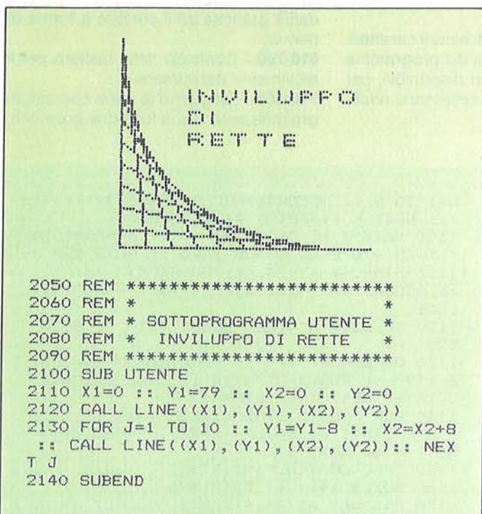
Figura 3 - Inviluppo di rette ottenuto con un ciclo For-Next nel quale viene chiamato il sottoprogramma Sub Line. Il testo è stato inserito controllando il cursore grafico con la tastiera. Infatti, creando una finestra in bit map non si dispone più del normale set di caratteri alfanumerici.
